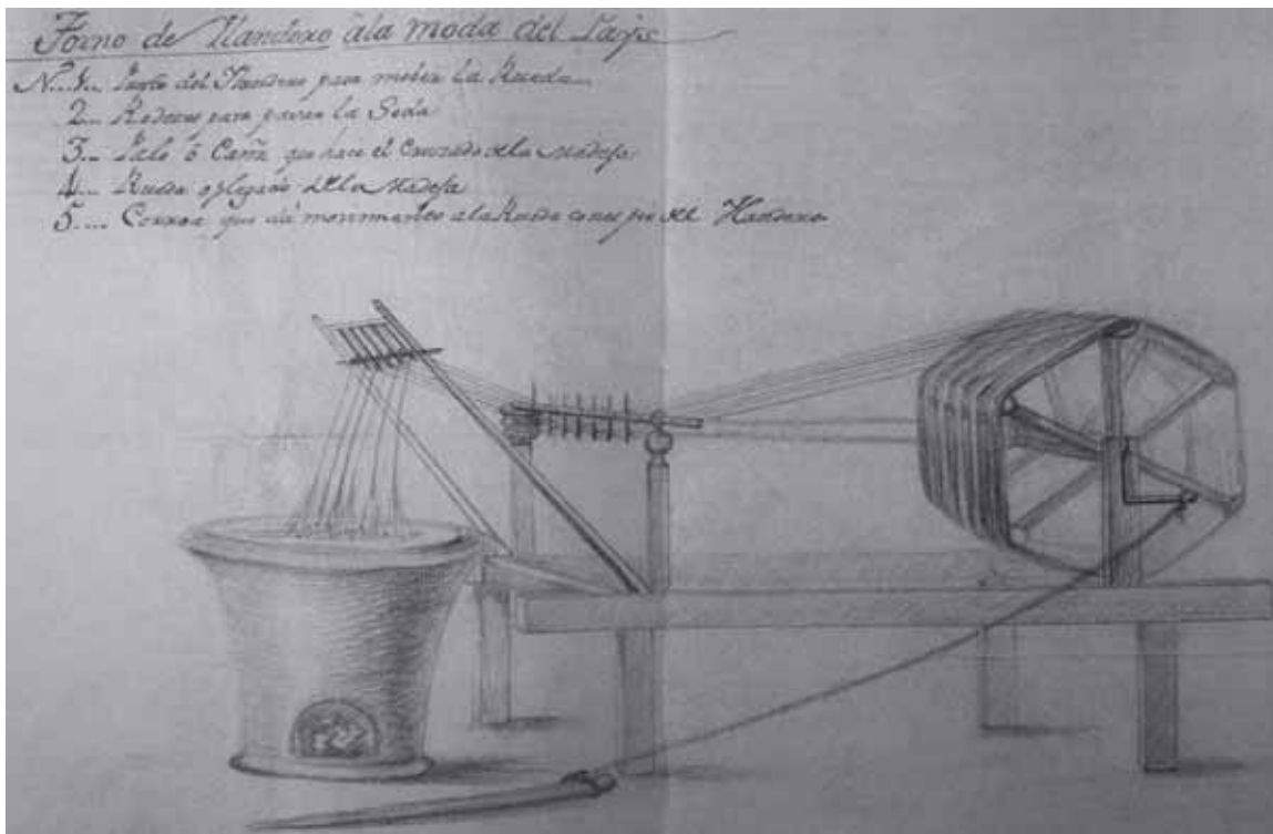
Torno de hiladero a la moda del Pays, Arte de hilar la seda . Dibujo de J. A. Valcárcel, RSEAPV
