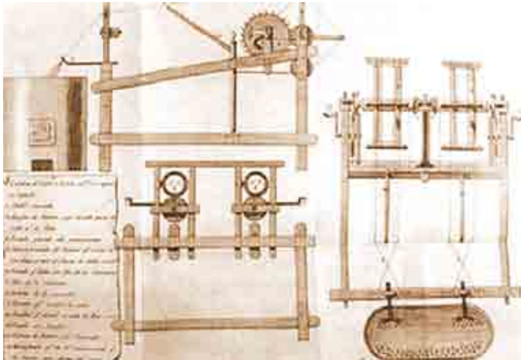
Torno doble de hilar seda instalado en la Fábrica de Lapayese en Vinalsa. Consiste en el torno de Jacques Vaucanson, mejorado por su discípulo Borceret y, a su vez, por el discípulo de éste llamado Toullet. Lo usaban dos hilanderas que utilizaban una sola caldera
