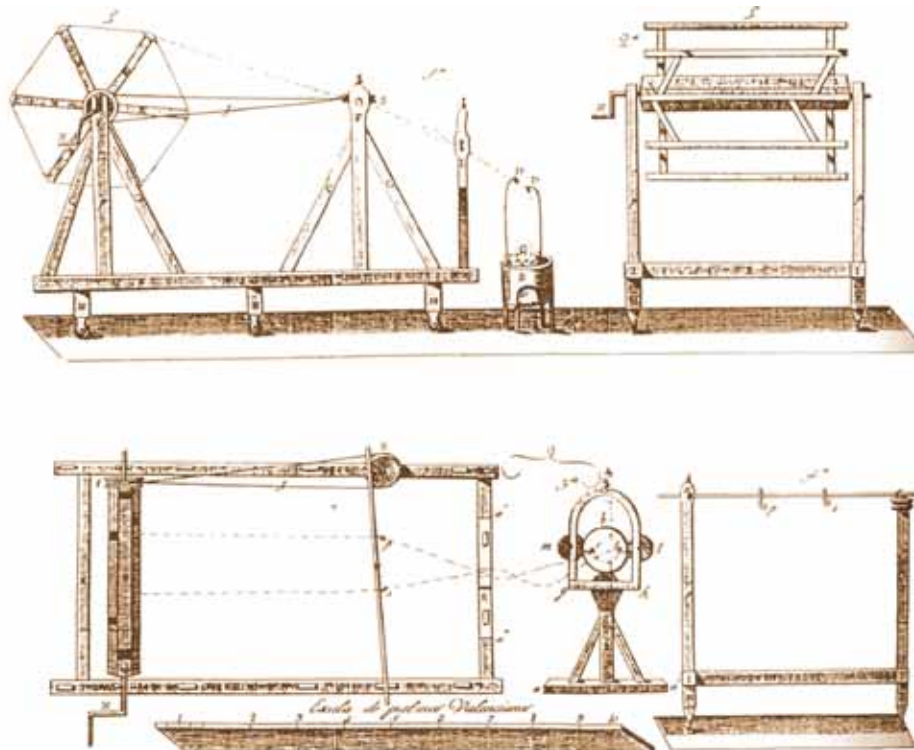
Torno inventado por el valenciano Vicente Taengua en 1821 cuando era director de la Fábrica de Vinalés
