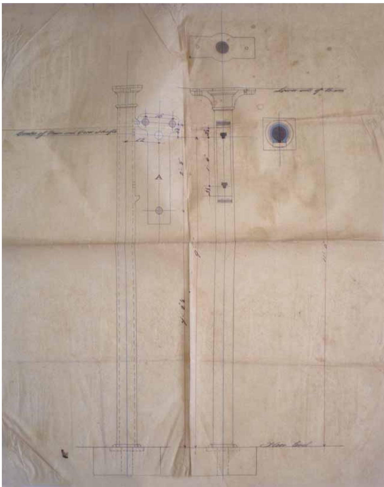
Eje de la rueda hidráulica instalada en el año 1853 en el cajero de la acequia de Montcada, para dotar de energía a la Fábrica (plano conservado en el Archivo Municipal de Vinalesa)
