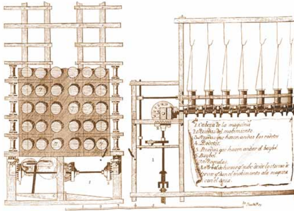
Máquina de doblar la seda mejorada por Toullot y adaptada por Lapayese a partir de un modelo ideado por Reboull
