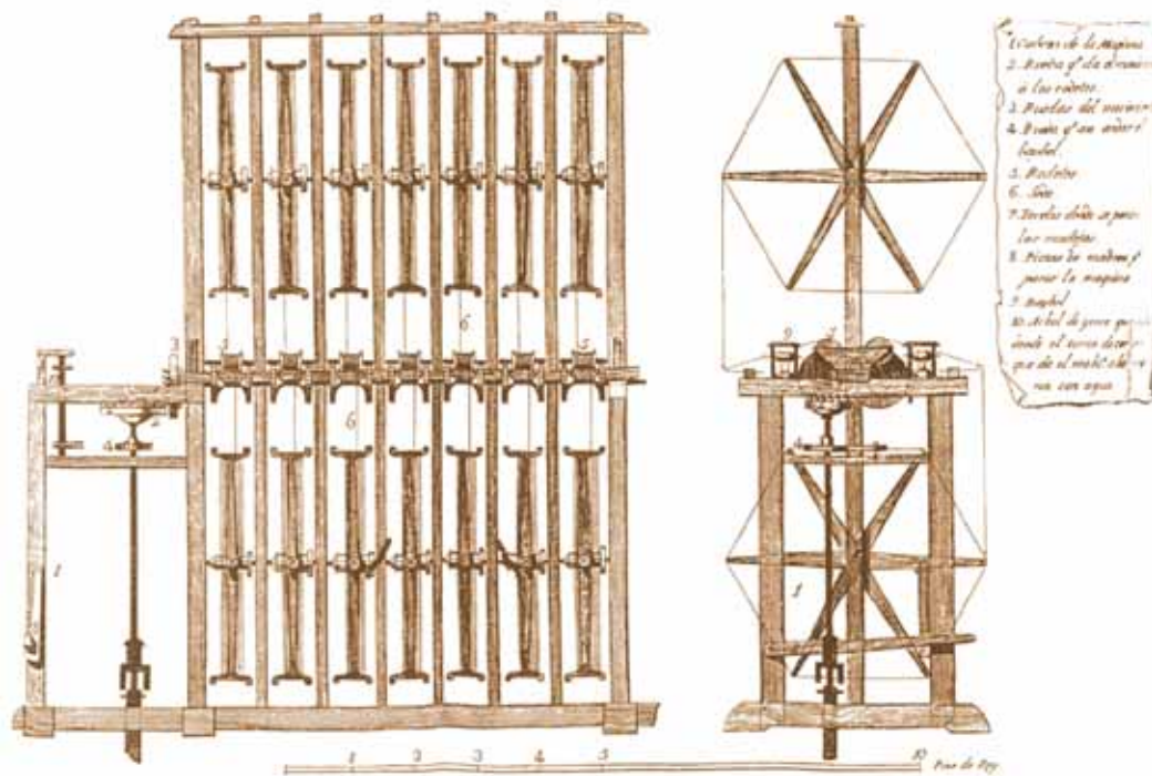
Devanadera de seda adaptada por Lapayese a partir del modelo de Vaucanson, introducido por Reboull y mejorado por Fco. Toullet. De menor tamaño, más ventajosa y sencilla en su manejo. Se componía de 70 tablillas o madejas
