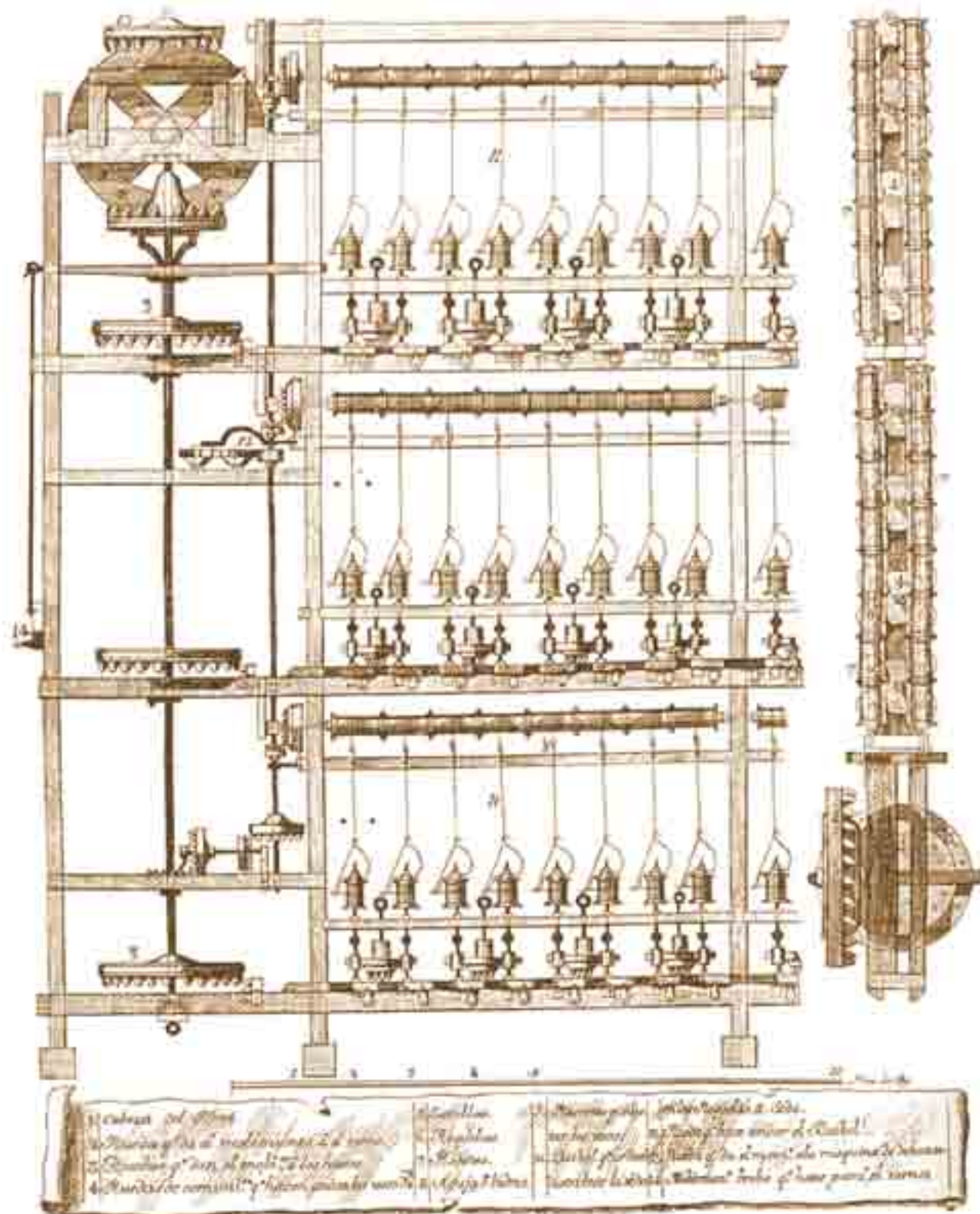
Torno de hilar Vaucanson, modificado por Francisco Toullot y Lapayese, utilizado en la Fábrica de Vinalés
