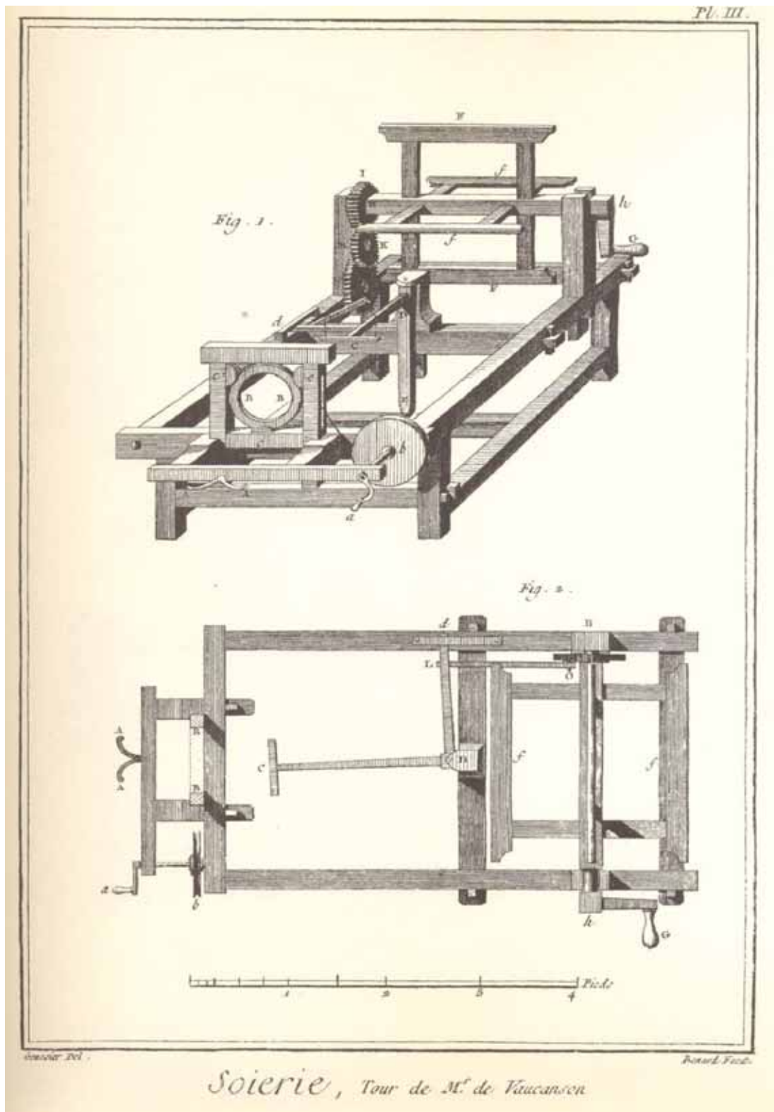
La enciclopedia de Diderot y D'Alembert refleja en esta ilustración el torno de hilar de Jacques Vaucanson, en ella se aprecian dos visiones diferentes: perspectiva y planta
