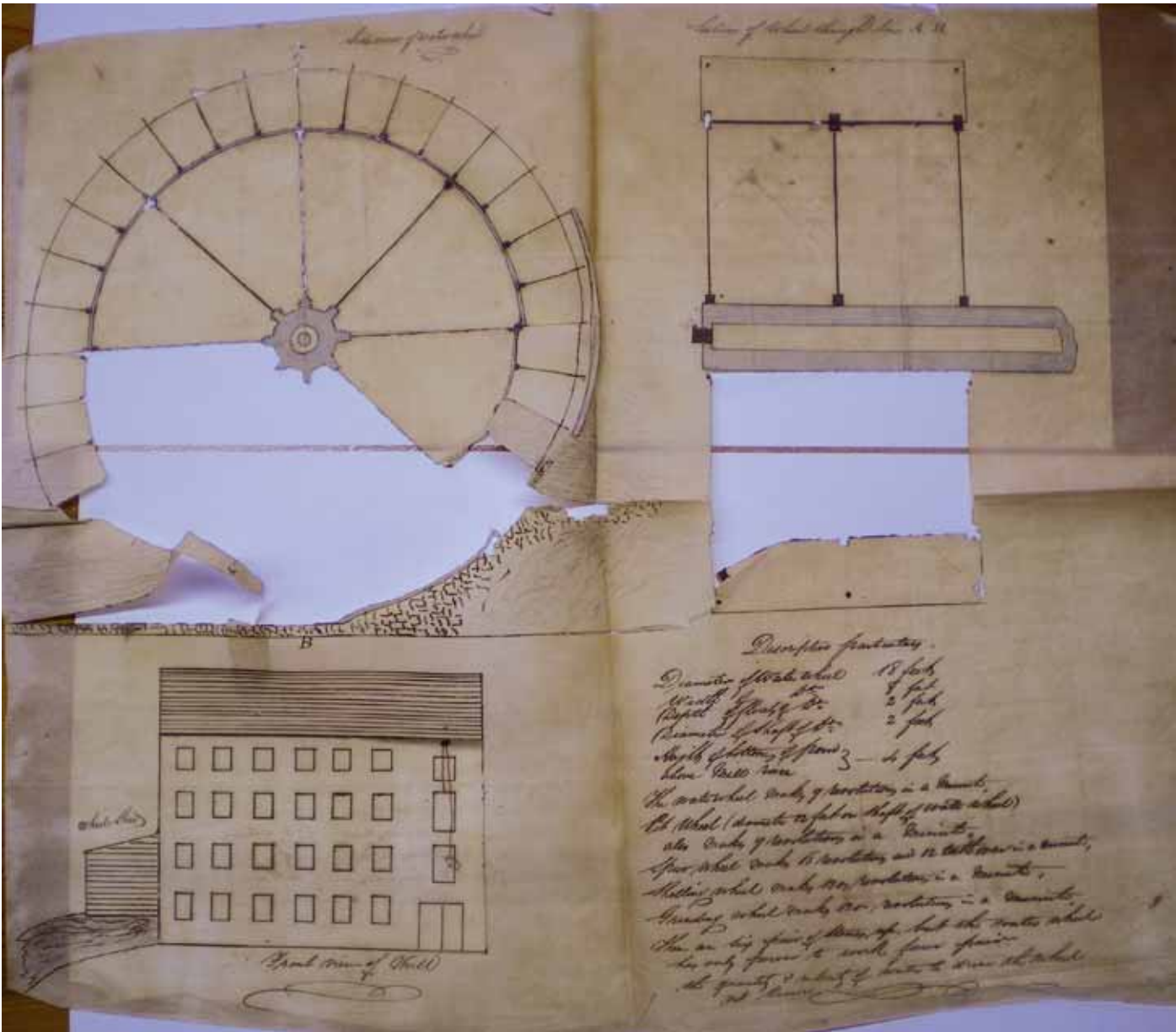
Plano muy deteriorado que se conserva en el archivo de Vinalés del diseño de la segunda rueda hidráulica que daba energía a la Fábrica, cuya instalación solicitó Tomás Trenor, el 27 de agosto de 1853, en el cajero de la acequia de Montcada
