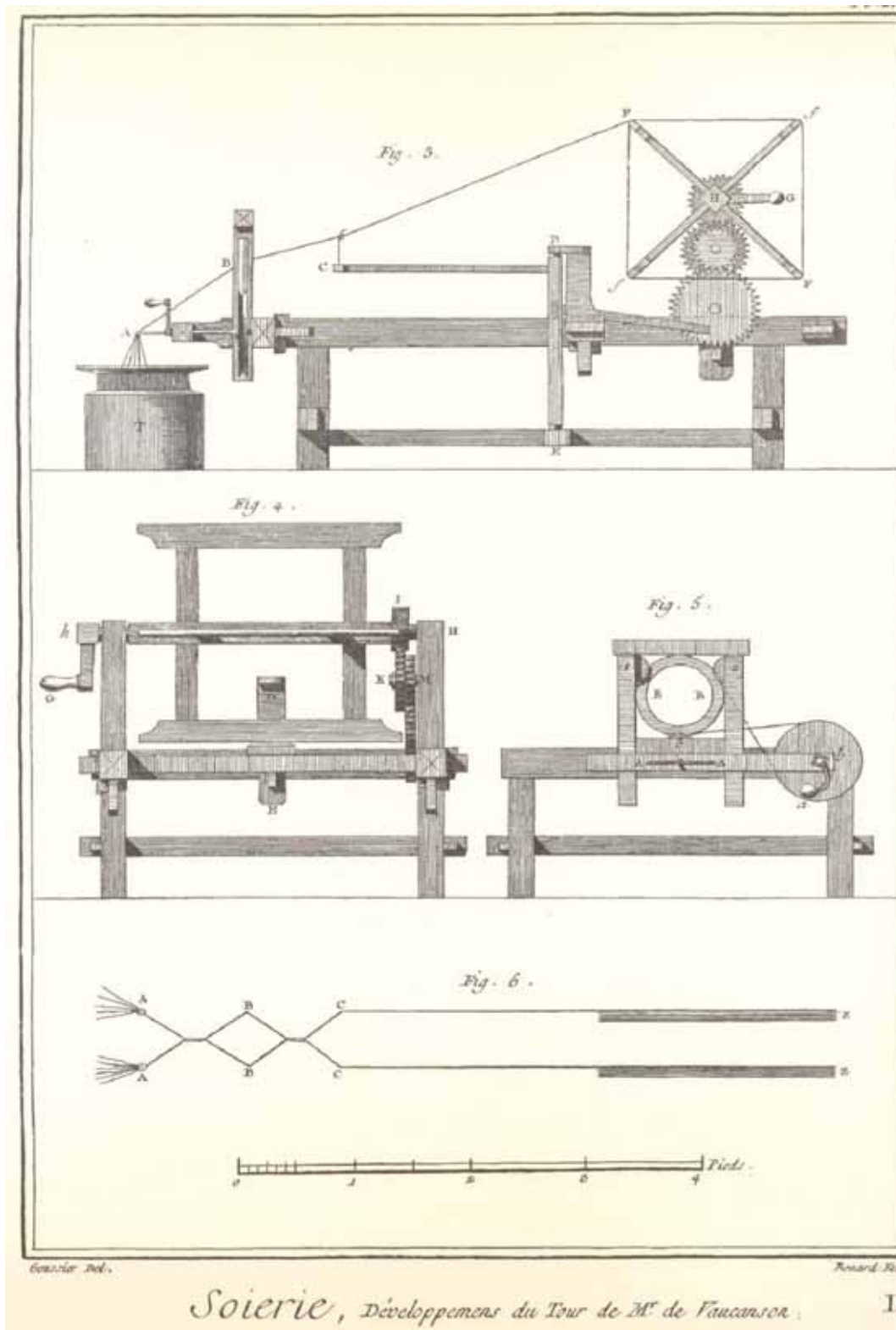
Enciclopedia de Diderot. En la ilustración se observa el torno de Jacques Vaucanson en un corte longitudinal, alzado desde la devanadera y desde la parte frontal
